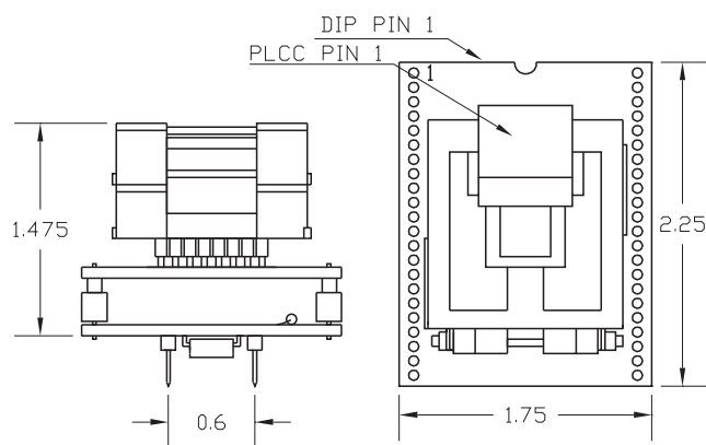
PA301-44Z(-A2)(-BP)(-LD)
