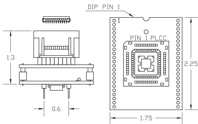
PA301-44(-A2)(-BP)(-LD)
